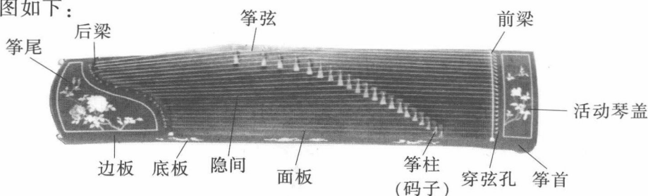
图 1 筝各部位名称(正面)
