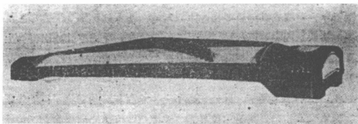
图8 营口二十一弦手板式转调筝
