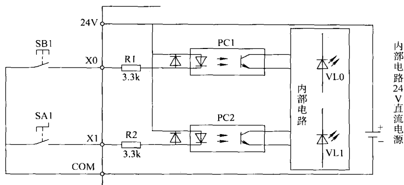
图 1-8 三菱 FX 系列 PLC 输入端子内部电路
