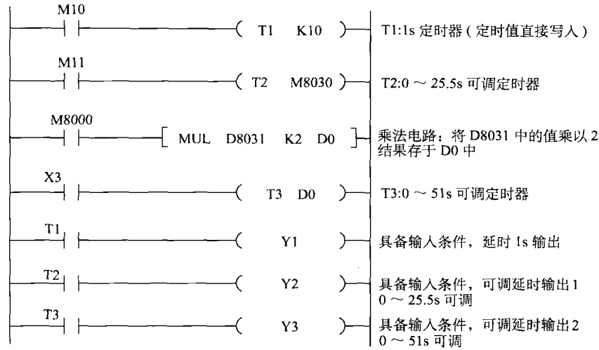
图 1-5 模拟电位器用于定时器时间调节的程序示例
