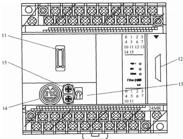
图 1-3 FX1N-24MR PLC 盖板打开图
