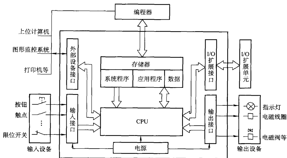
图 1-1 PLC 的典型电路结构图
