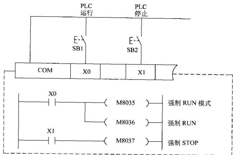
图 1-4 用程序及输入端子控制 PLC RUN/STOP
