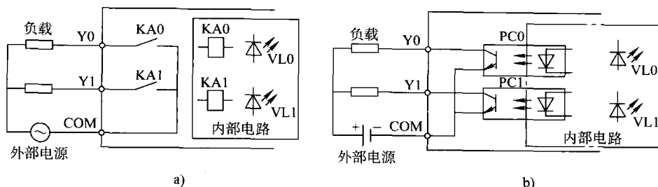
图 1-10 三菱 FX1N 系列 PLC 两种输出电路
