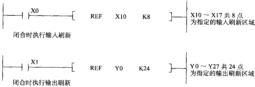
图 1-11 I/O 刷新指令程序示例
