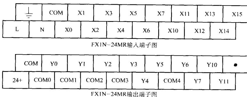
图 1-6 FX1N-24MR PLC 端子标记
