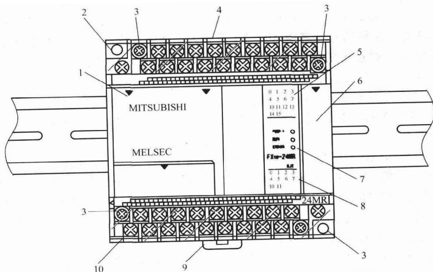
图 1-2 FX1N-24MR PLC 外形
