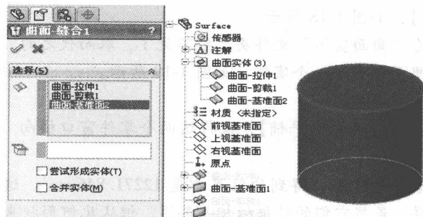
图 1-16 缝合曲面
