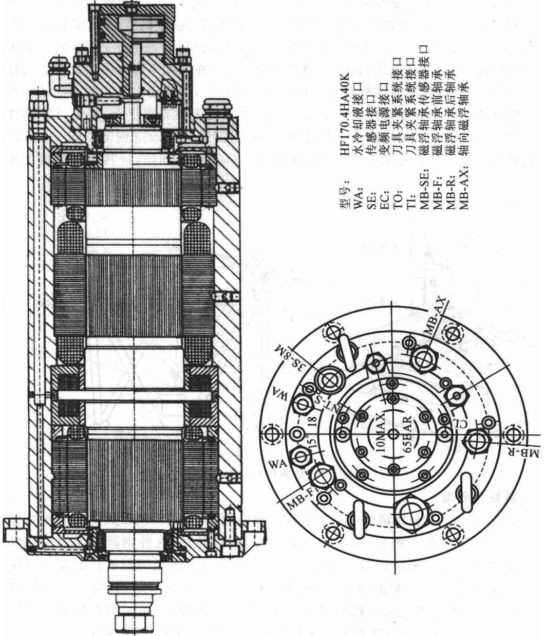
图 1-4 具有磁悬浮轴承的电机轴结构
