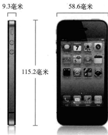
图1.3 iPhone 4尺寸
