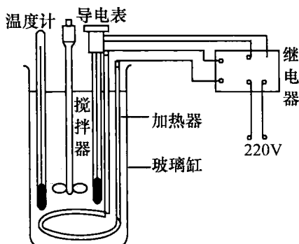
图 4 恒温装置组装简图
