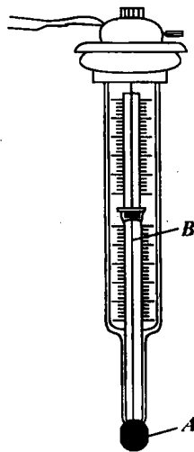
图 2 水银接点温度计型温度控制器
