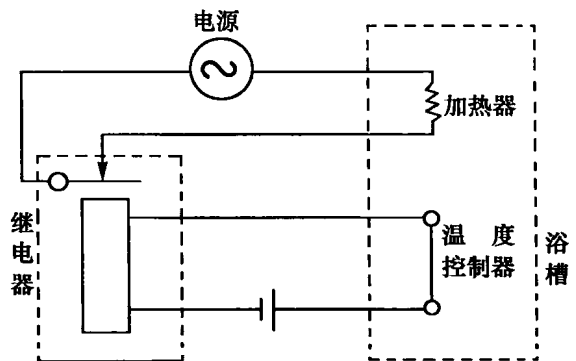
图1 恒温装置示意图
