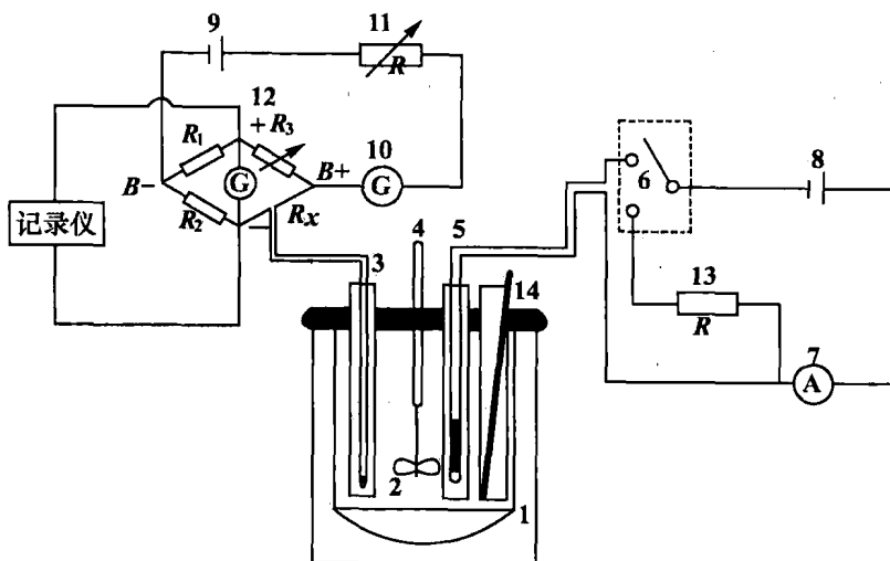
图 1 量热实验装置简图
