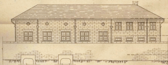
南面立视图
