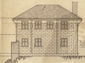
东面立视图
