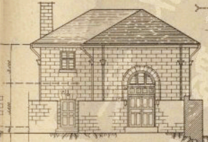
西面立视图
