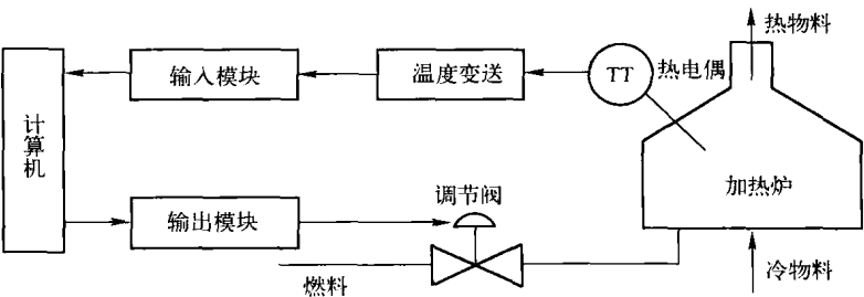
图 1-3 计算机温度控制系统
