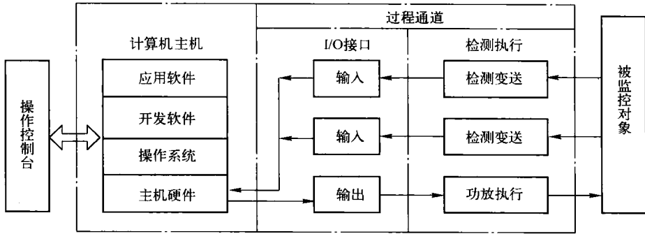
图 1-5 计算机控制系统组成原理简图
