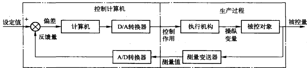
图 1-2 计算机控制系统典型结构框图
