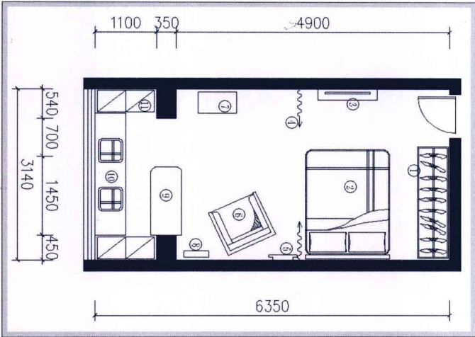
改造后平面布置图
