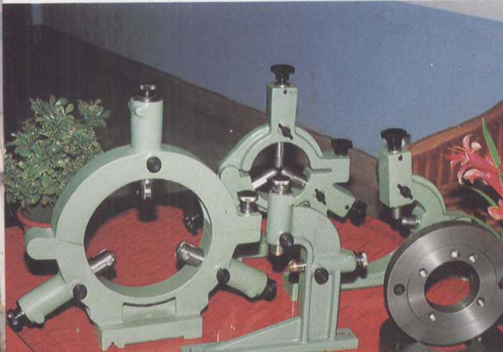
▼ 机械厂生产的 66140 型机床中跟架
