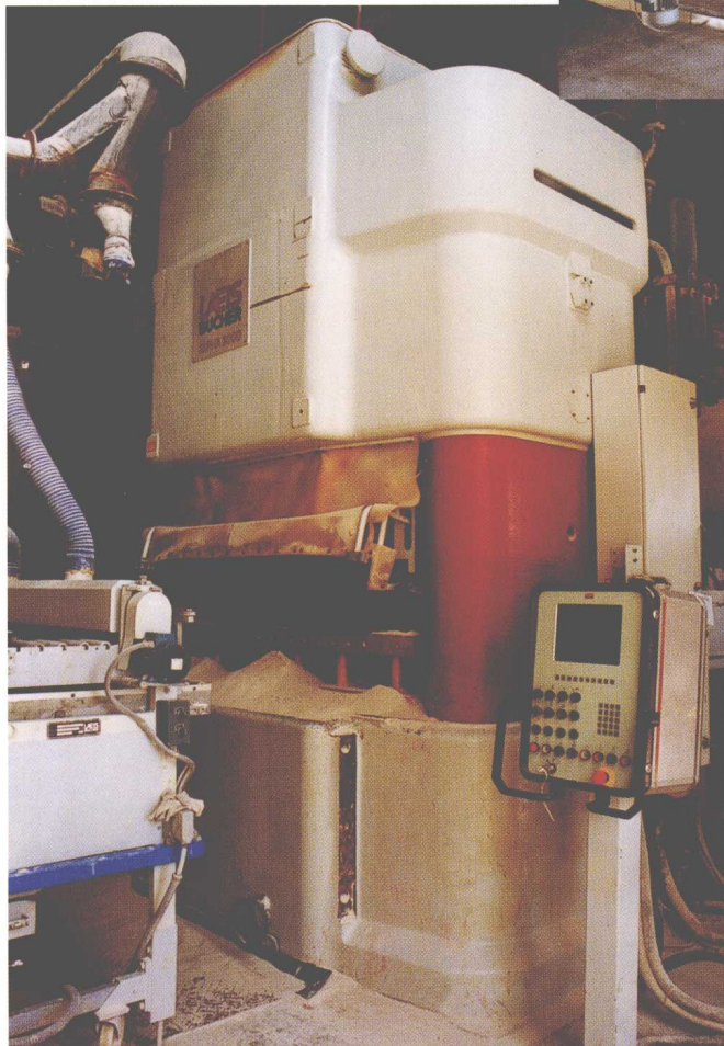
高安市高峰陶瓷集团 公司玻化砖压力成型机
