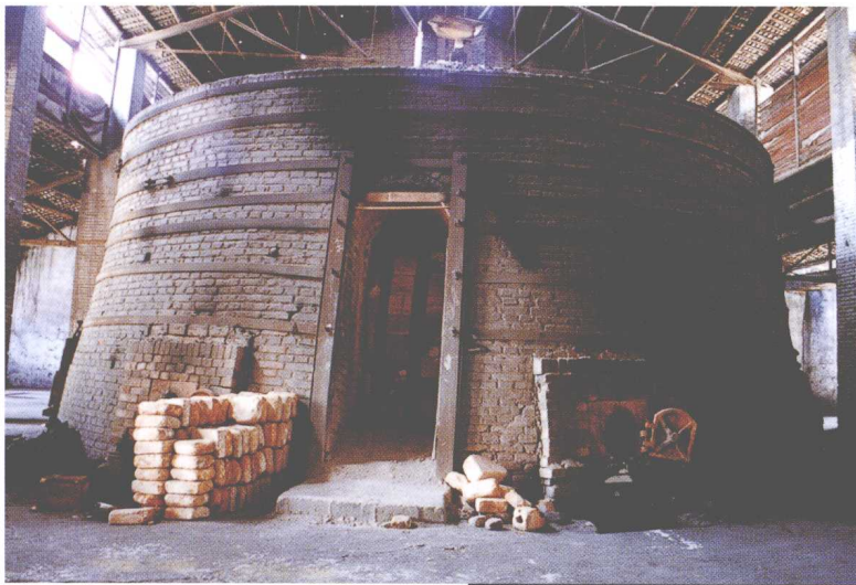
高安市石脑陶瓷厂老式圆堡窑
