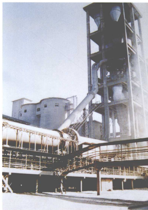
南昌水泥厂日产 700 吨 熟料窑外分解生产线
