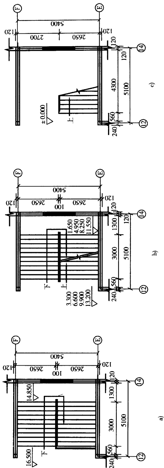
图1-8 建施8楼梯2平面图 (单位:mm)
