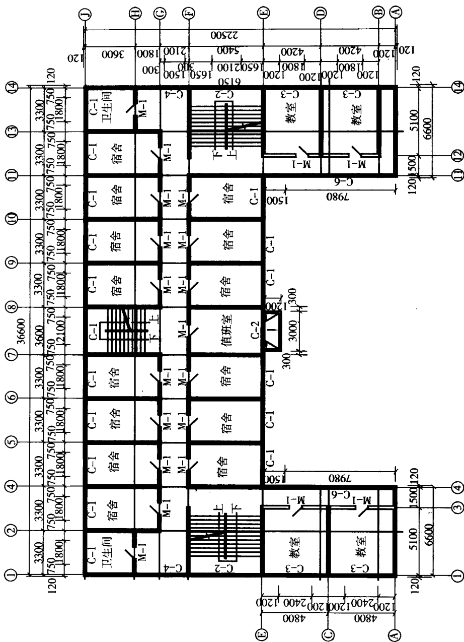
图1-2 建设2标准层平面图 (单位:mm)
