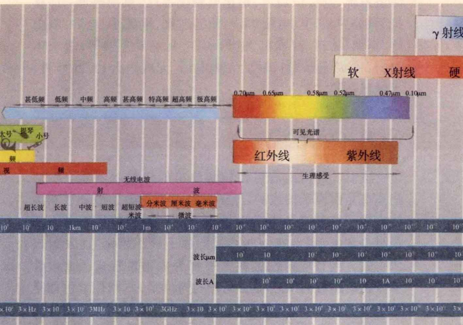
电磁波频谱
