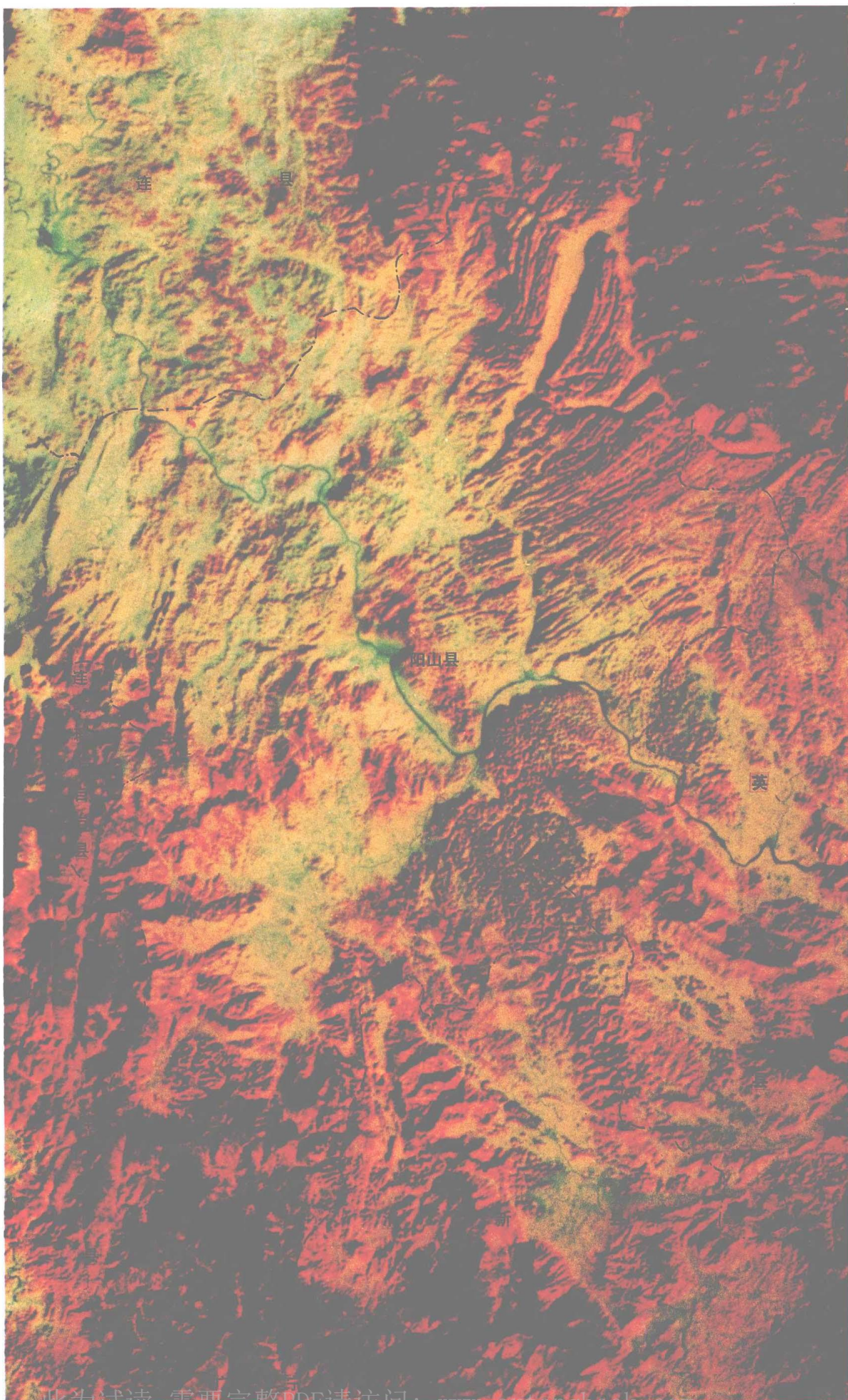
阳山县卫星影像图 (比例尺 1:430000)
