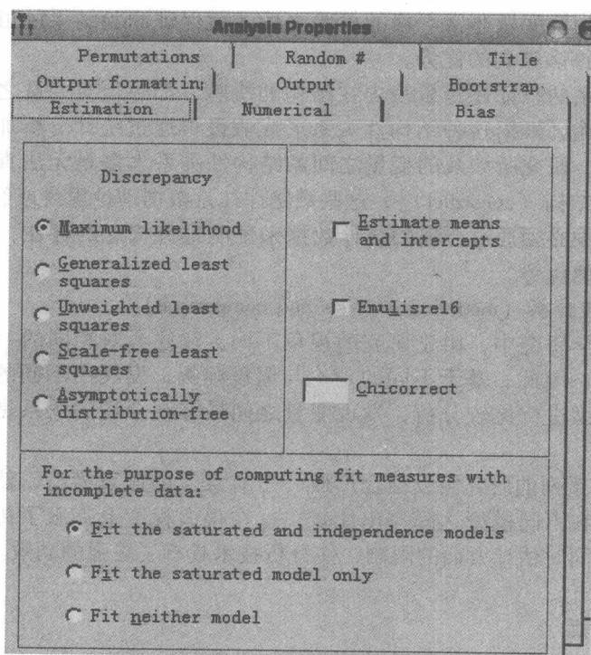
图 1 - 1 AMOS 的估计方法设置窗口
