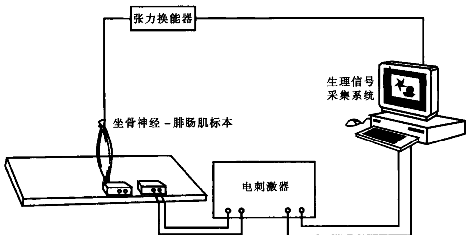
图 2-1 骨骼肌单收缩和复合收缩实验装置连接示意图
