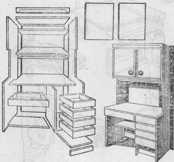
图 1-5 板式家具的板块组装结构
