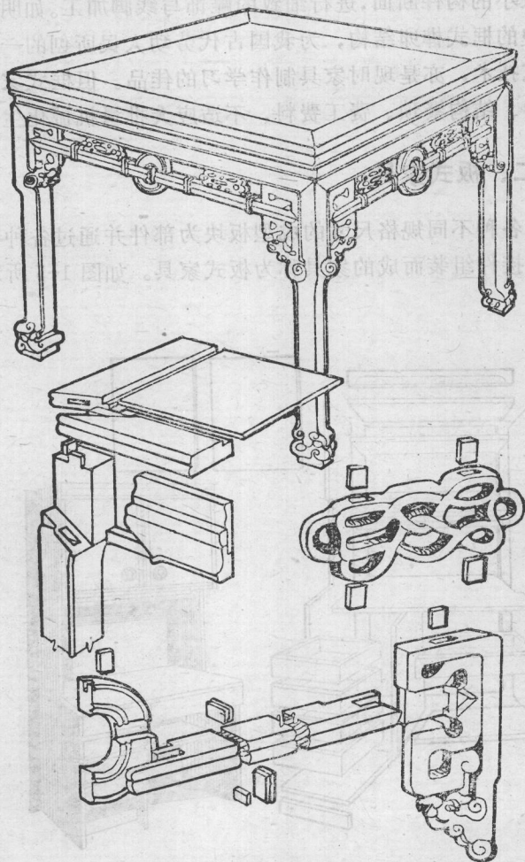
图 1-4 框架式家具的榫卯结构
