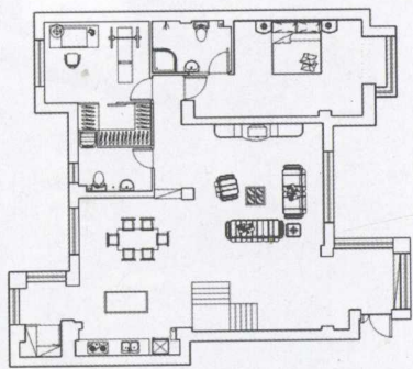
✧ 一层平面图
