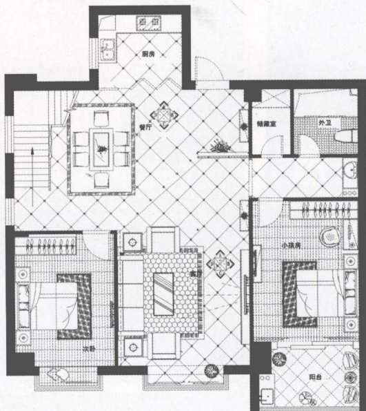
※ 一层平面布置图
