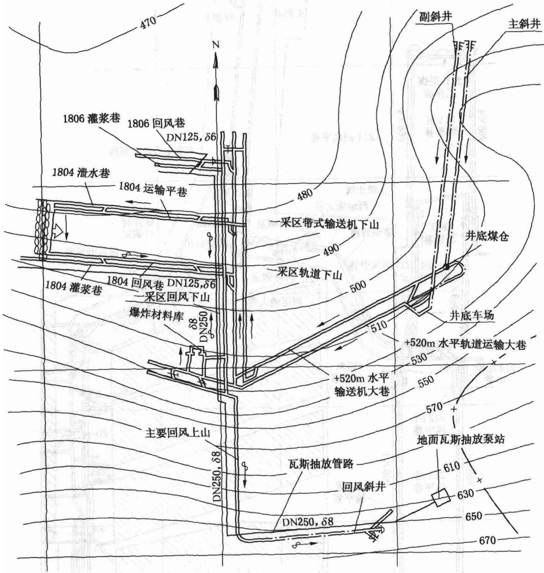
图 1-3 某矿瓦斯抽放管路系统平面图
