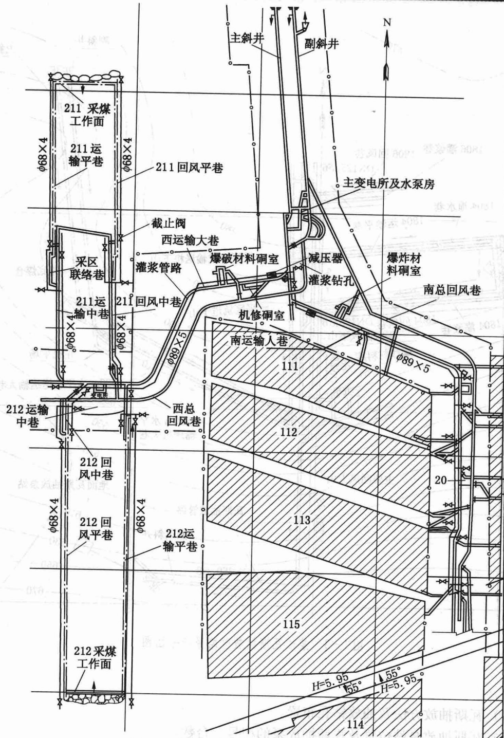
图 1-2 某矿井黄泥灌浆管路系统工程平面图
