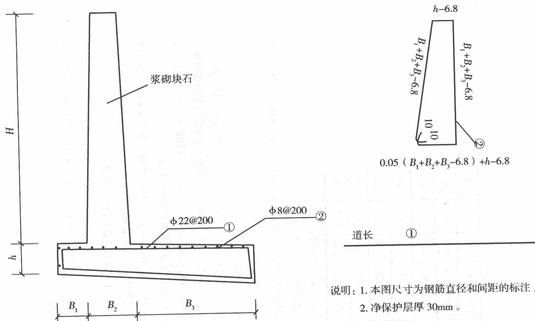
图 1-6 挡土墙配筋示意图
