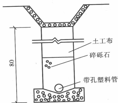
图 1-9 1号道路盲沟构造示意图
