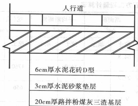
图 1-11 2 号道路人行道结构示意图
