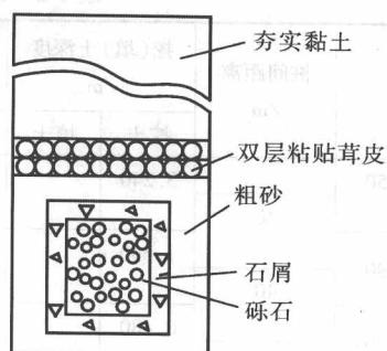
图 1-12 2 号道路盲沟构造示意图
