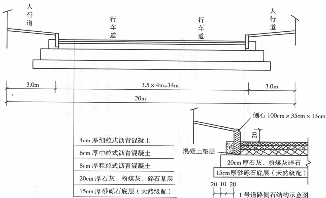
图 1-2 1 号道路路面结构示意图
