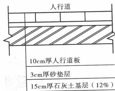
图 1-8 1号道路人行道结构示意图
