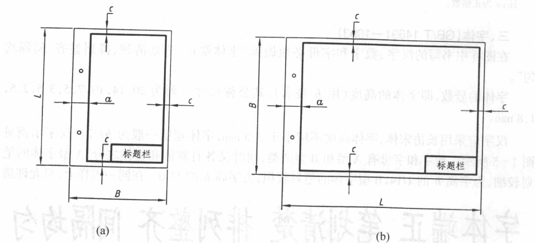
图 1-3 留有装订边的图框格式
