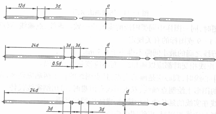
图 1-9 图线的构成
