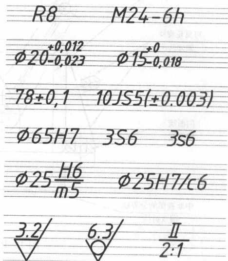
图 1-8 字体综合运用示例
