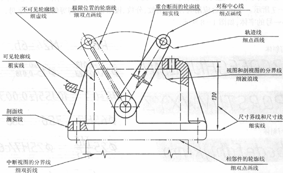
图 1-10 图线的应用示例
