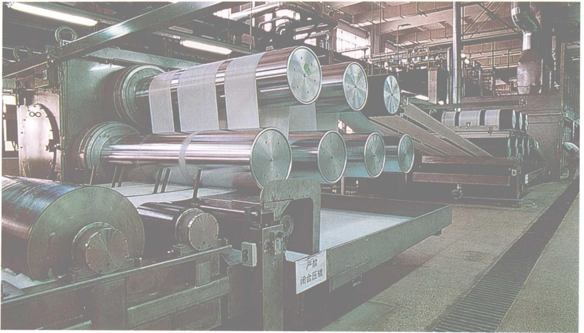
化纤厂16万吨/年直接纺涤纶短纤维生产线
