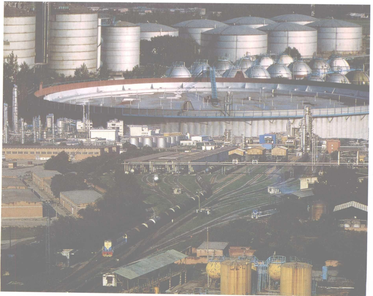
▽ 洛阳石化总厂储运分厂主要设施
