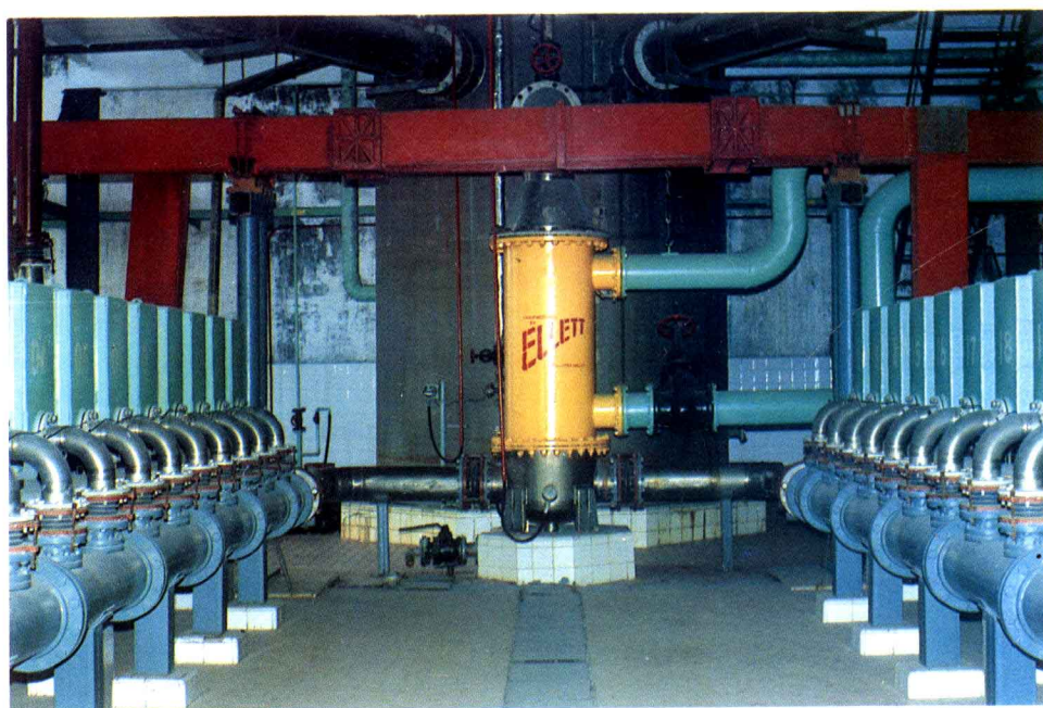
福州第一化工厂引进芬兰诺基亚化学公司1万吨/年氯酸盐电解槽装置
