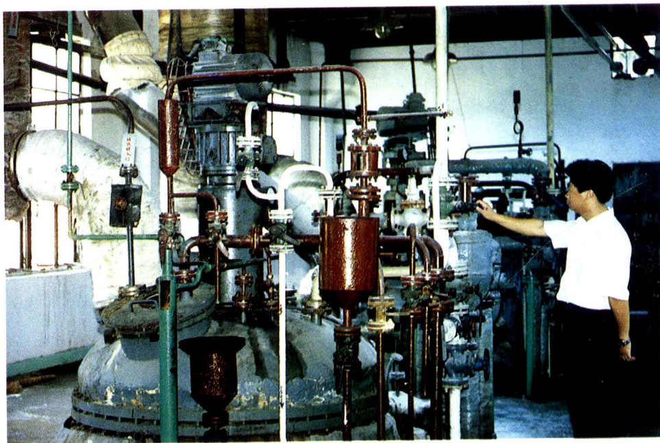
福州医疗化工总公司 5000 吨 / 年增塑剂生产装置
