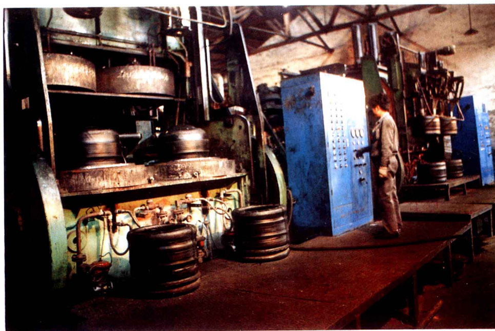
福州橡胶厂轮胎自动定型硫化装置
