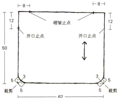
袋布 2 片
