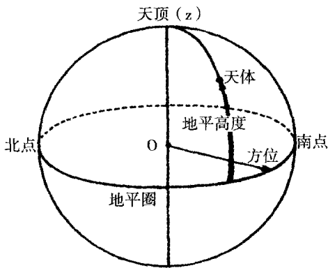
图1 地平坐标系
