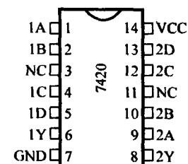
74H21、74F21、74ALS21、74LS21、74HC21 双 4 输入与门
