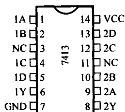
7414、74LS14、74HC14、74C14 六反相器（施密特触发）
