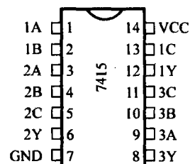
7416、74LS16 六反相缓冲器/驱动器（OC、高压输出）
