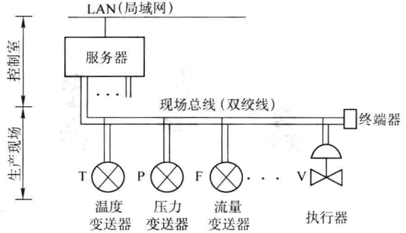
图 1-8 现场总线数字仪表一对多连接
