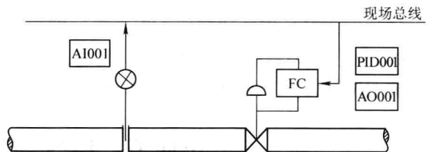
图 1-9 由现场总线数字仪表实现流量控制
