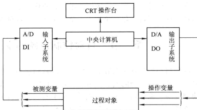
图 1-2 DDC 的结构图
