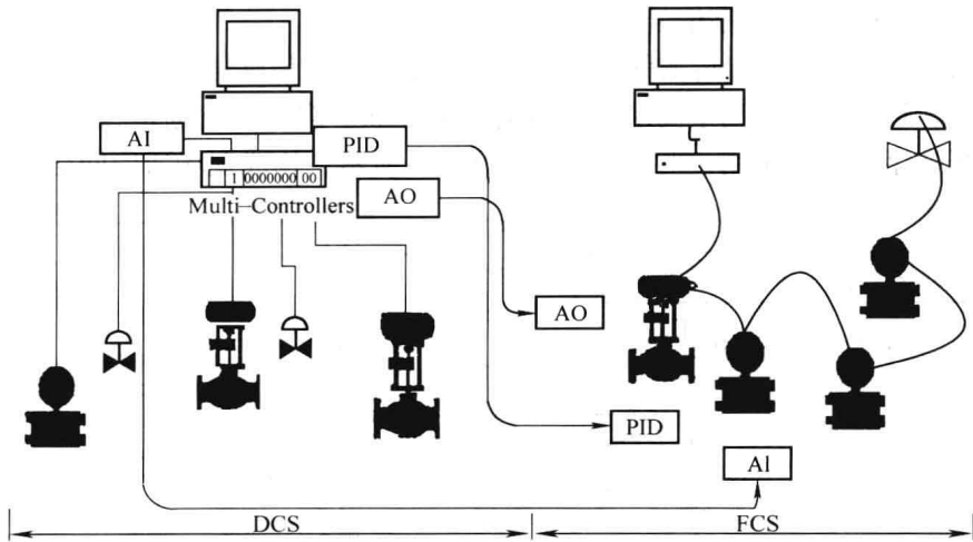
图 1-6 现场总线控制系统与传统控制系统的结构对比
