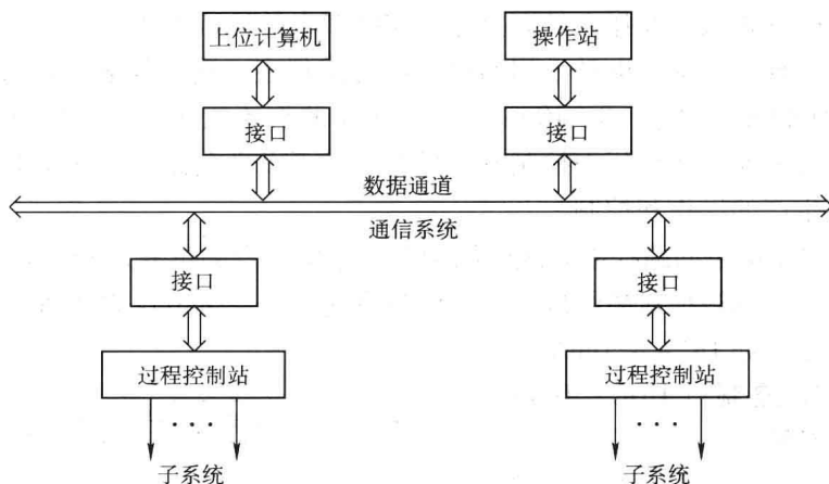
图 1-3 典型的 DCS 结构图
