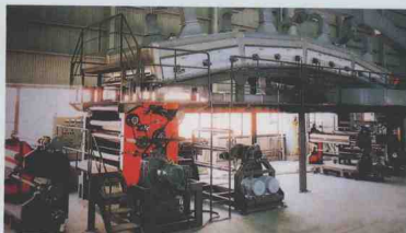
TB-650 1300型凹輥（離型逆轉）塗布機
