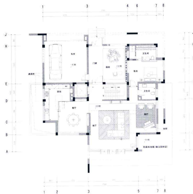
一层平面布置图
