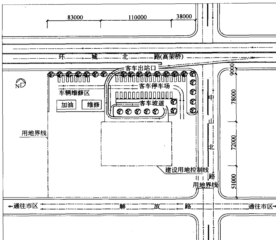
图 1-1 总平面图 1 : 2500
