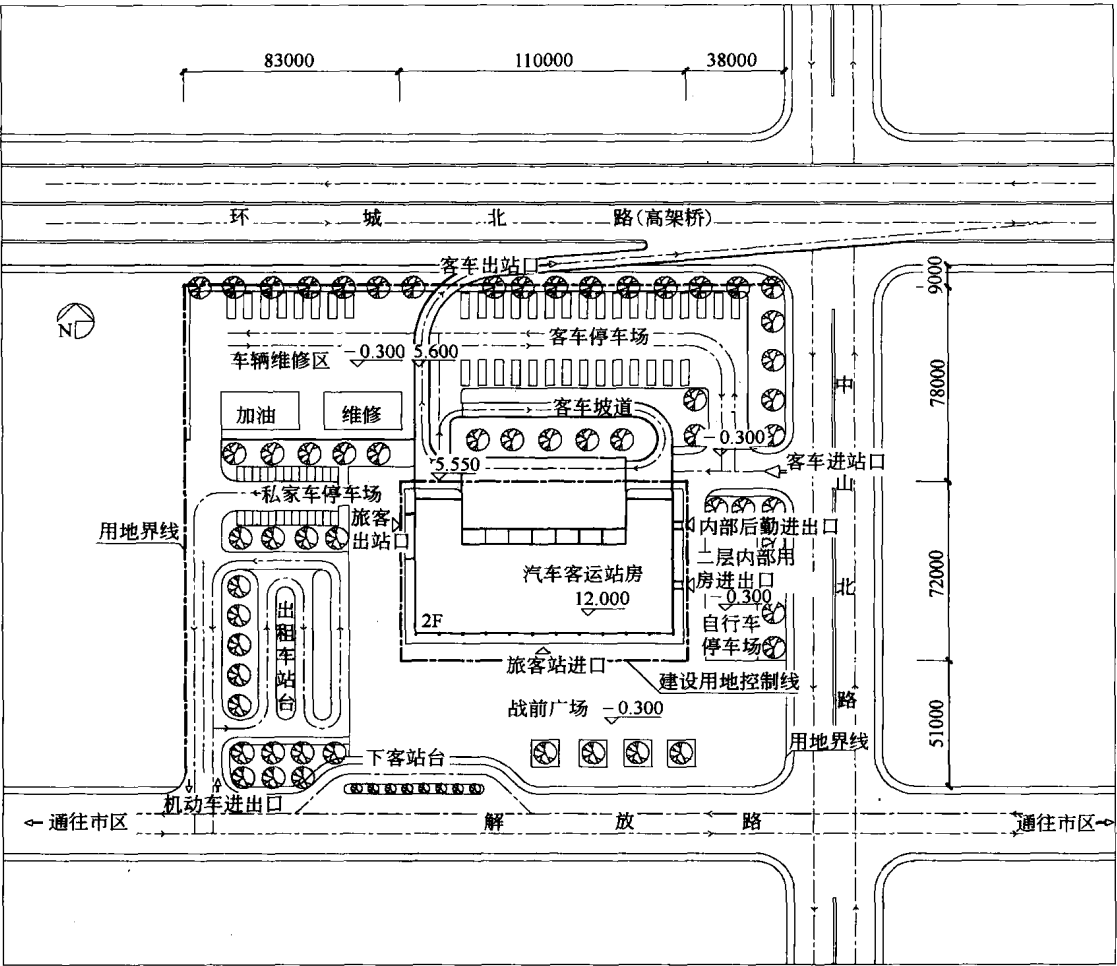
图 1-7 总平面 1 : 2500
