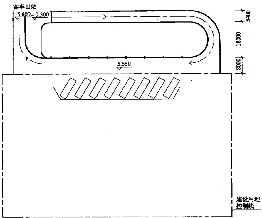
图 1-3 二层平面图 1 : 800
