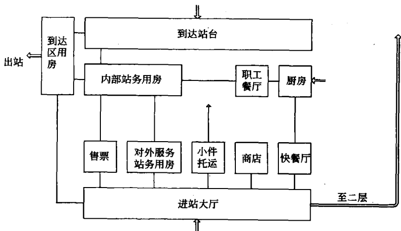
图 1-5 一层主要功能关系图
