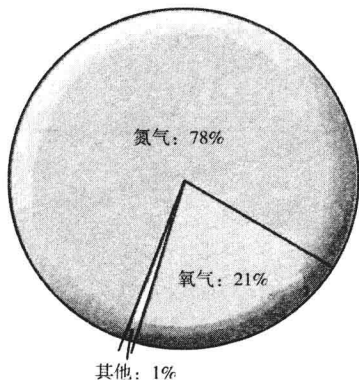
◆地球大气成分图
