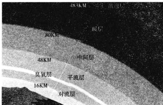
◆大气层结构
