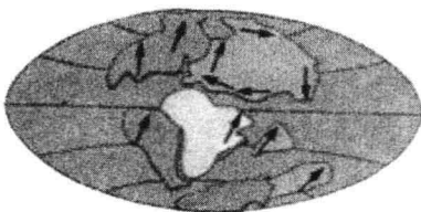
1亿3500万年前（白垩纪初）
