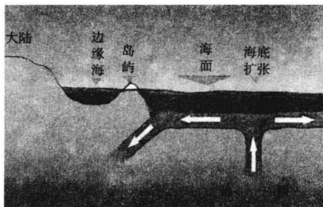
◆海底扩张形成海沟示意图
