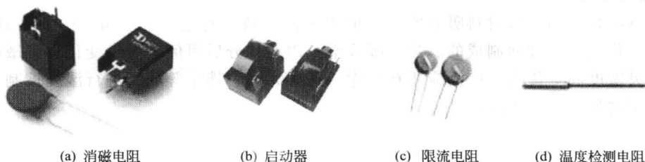
图 1-5 常见的热敏电阻实物示意图
