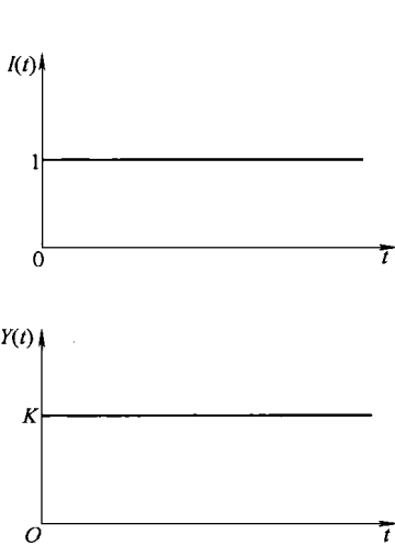
图 1-10 零阶传感器的单位阶跃响应
