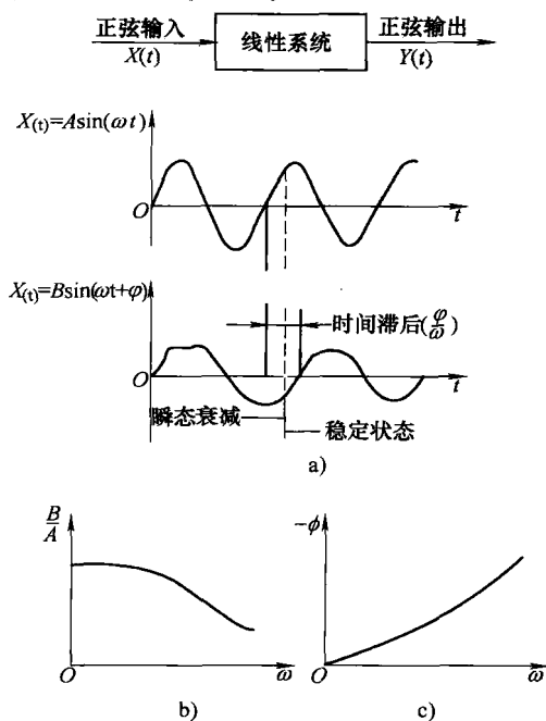
图 1-9 正弦输入的频率响应
