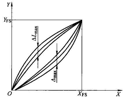
图 1-6 传感器的重复性
