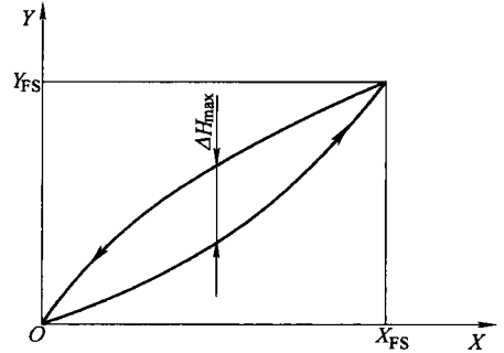
图 1-5 传感器的迟滞特性
