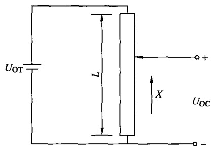
图 1-7 零阶传感器
