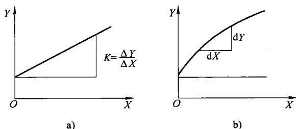
图 1-4 传感器灵敏度的定义 a) 线性传感器 b) 非线性传感器
