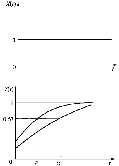
图 1-11 一阶传感器的阶跃响应
