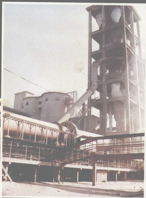
南昌水泥厂日产700吨熟料的旋风预热器窑外分解窑
