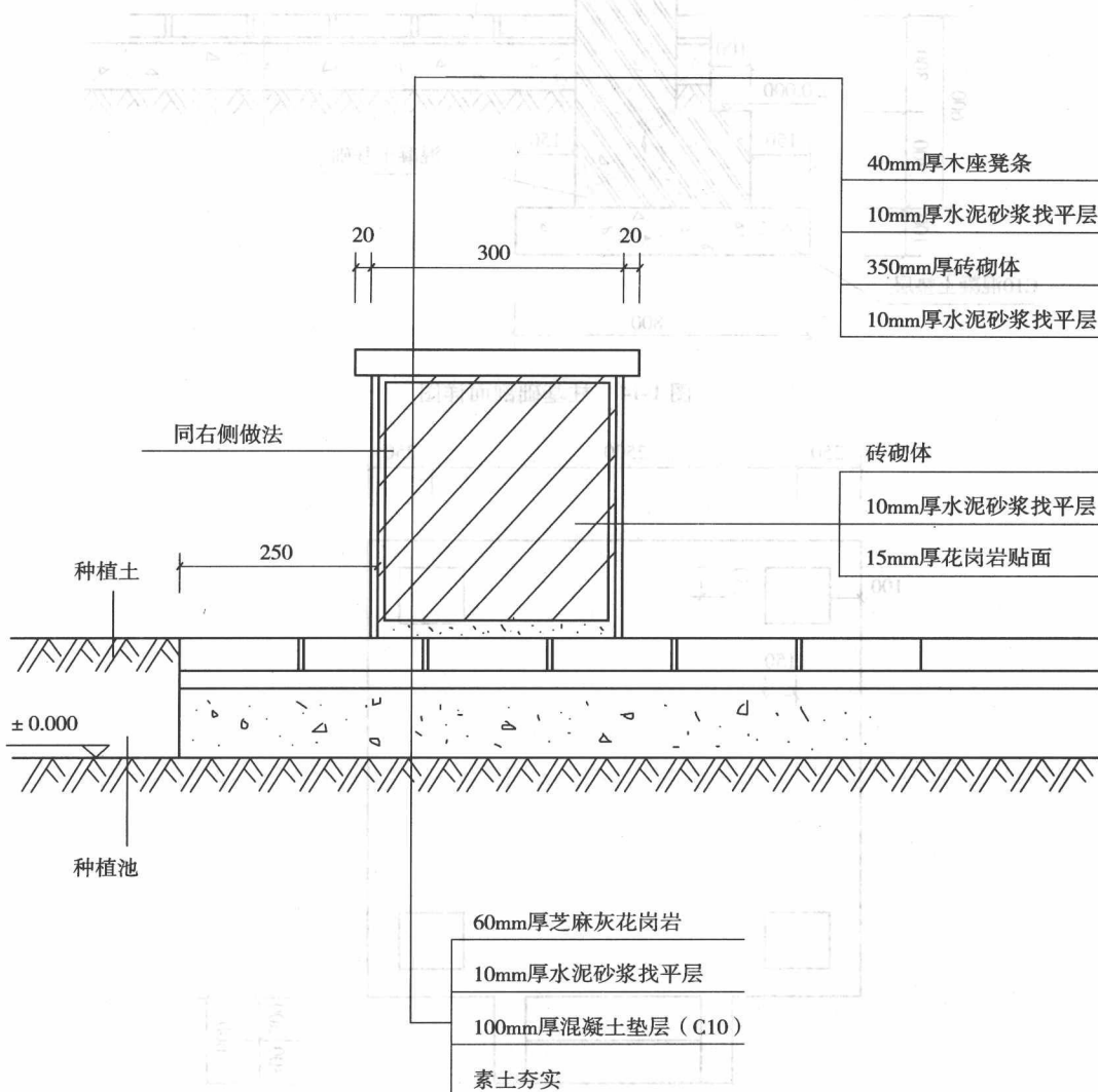
图 1-13 座凳剖面大样
