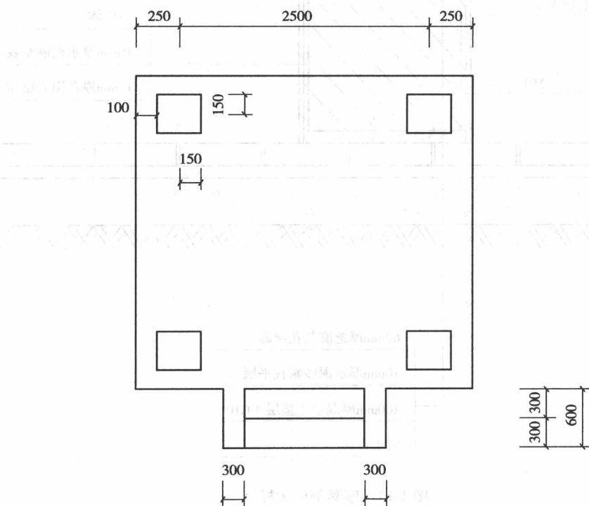
图 1-15 柱基础平面图
