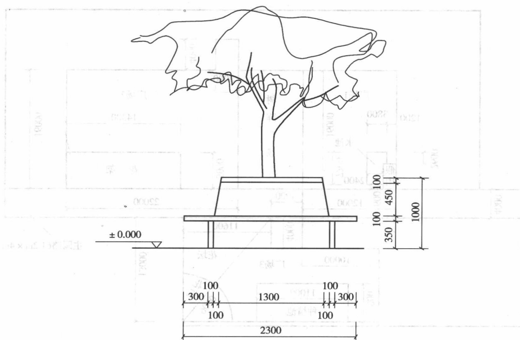
图 1-10 围树椅立面图
