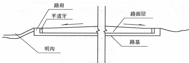
图 1-6 平道牙示意图
