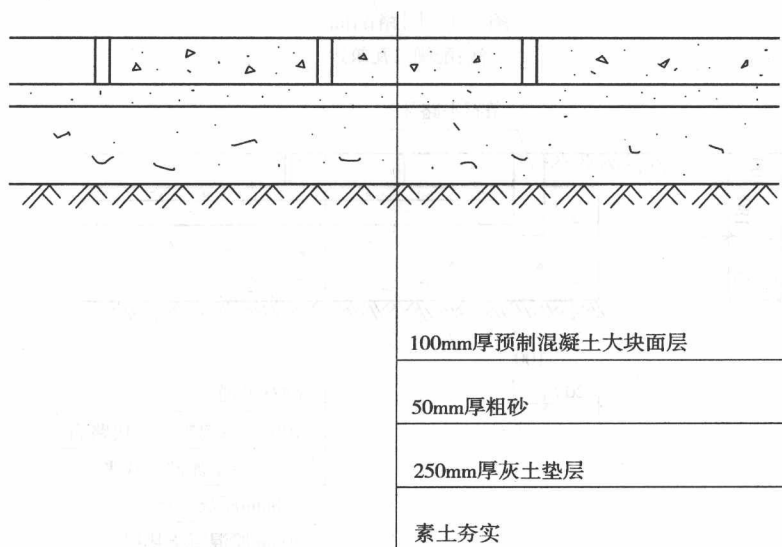
图 1-7 广场剖面示意图
