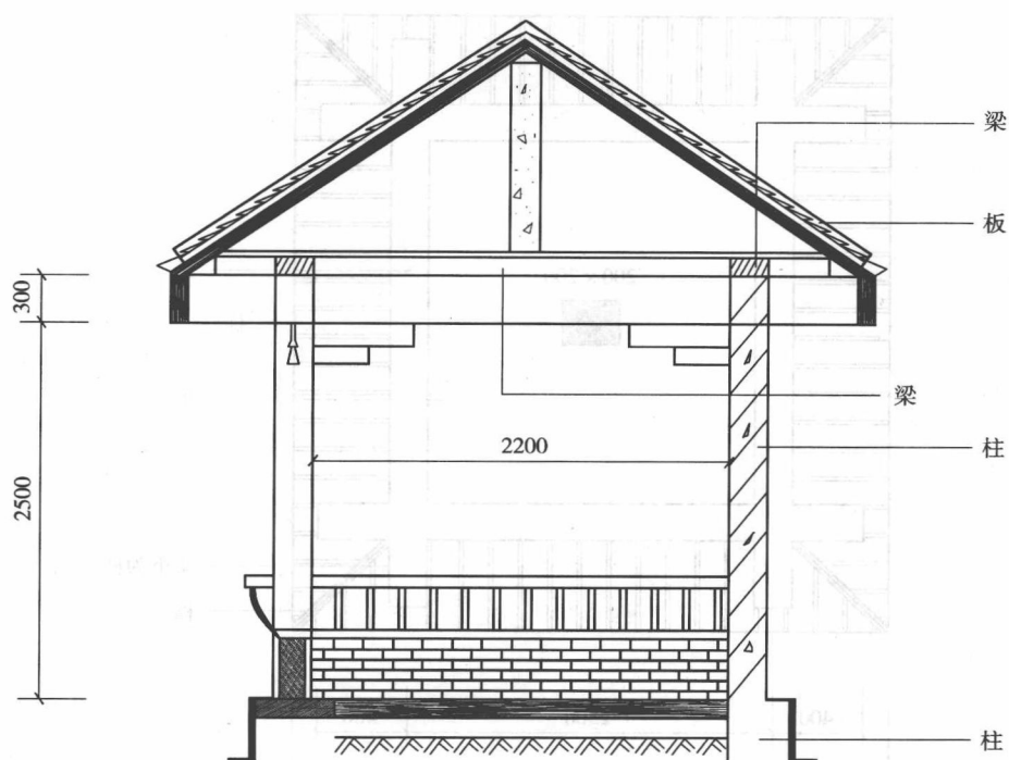
图 1-18 剖面图
