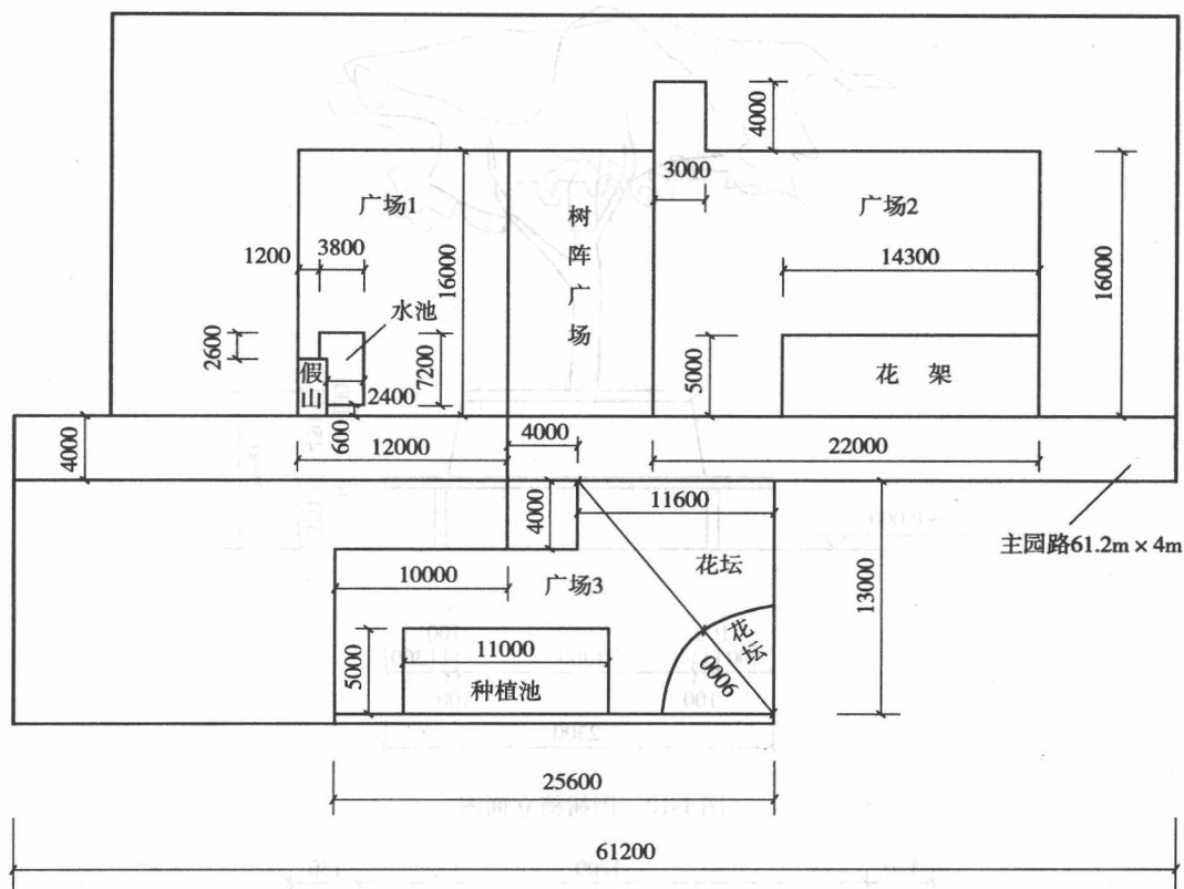
图 1-8 平面尺寸详图
