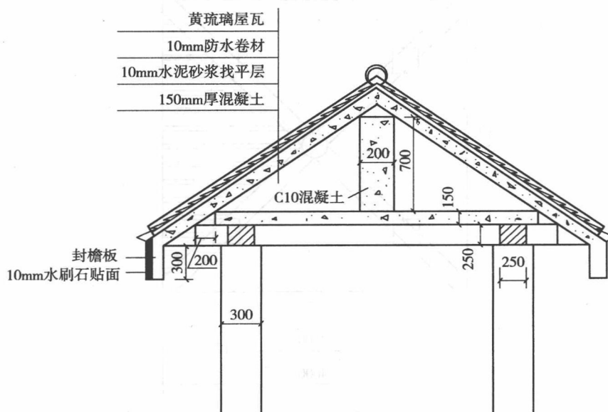
图 1-17 屋顶剖面详图
