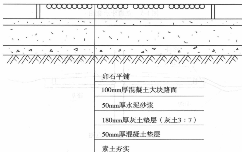
图 1-3 园路剖面图
