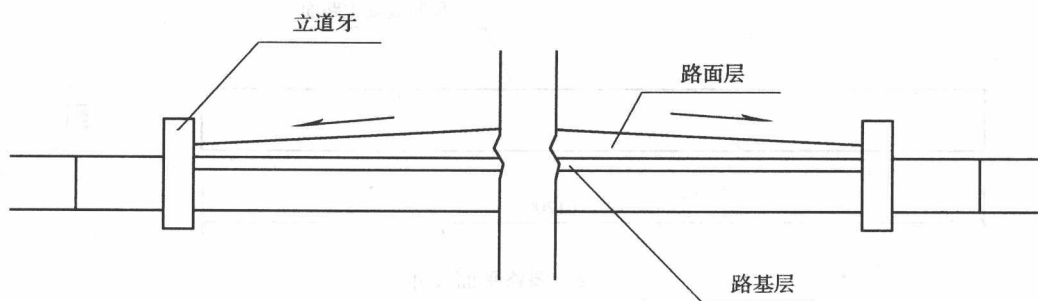
图 1-5 立道牙示意图
