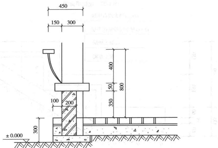
图 1-21 座椅剖面图
