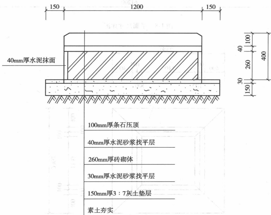
图 1-11 座凳剖面图
