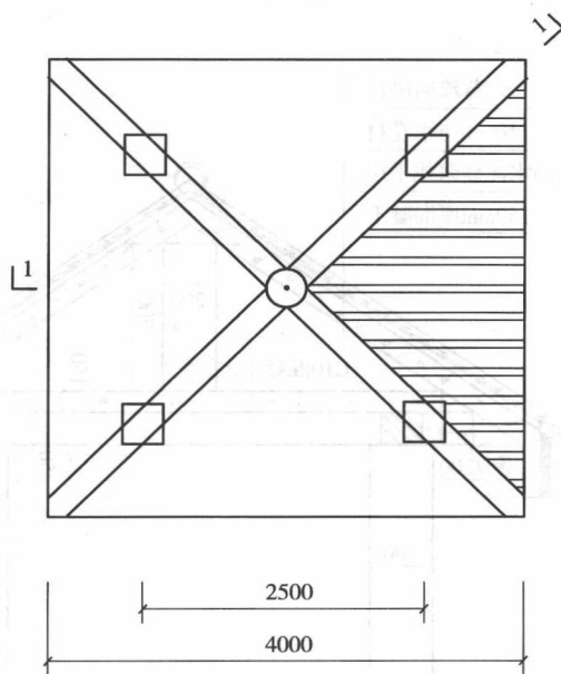
图 1-19 屋顶平面图
