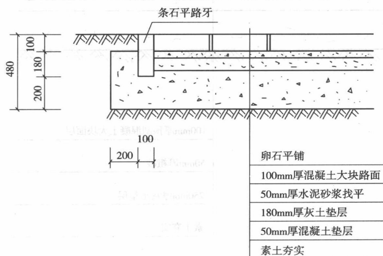
图 1-4 条石平路牙及路面详图
