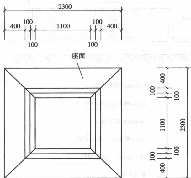
图 1-9 围树椅平面图
