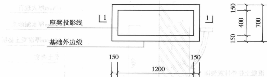
图 1-12 座凳基础平面图
