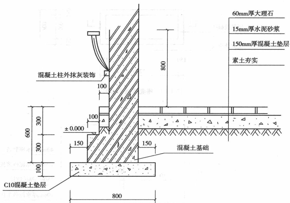
图 1-14 柱基础剖面详图
