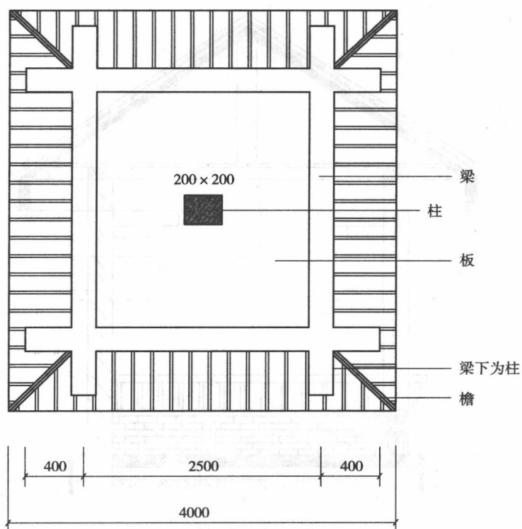
图 1-16 亭顶剖面图 2-2'
