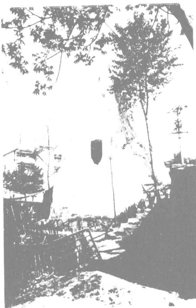
地质钻探
