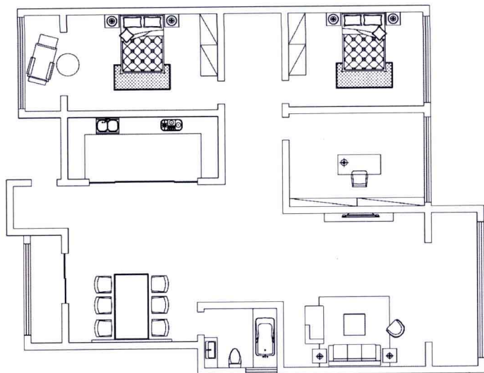
※ 平面布置图
