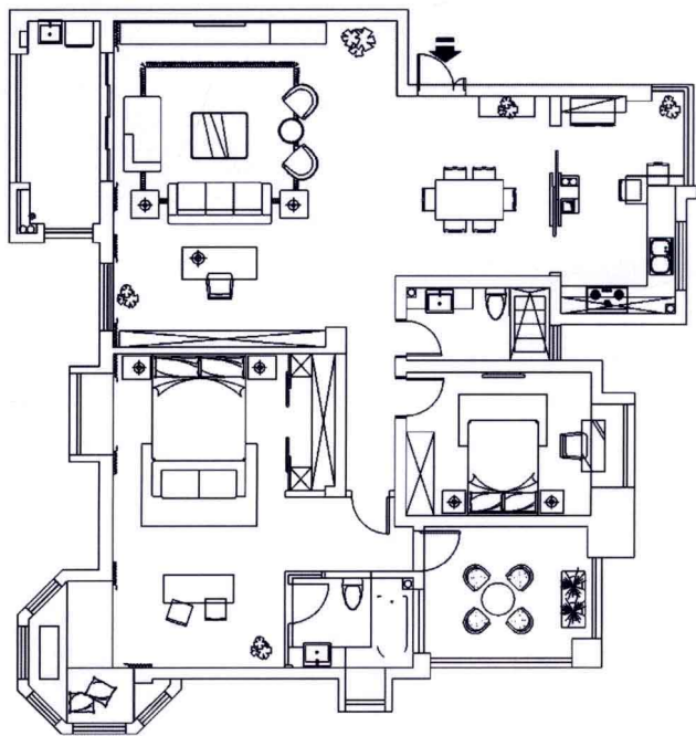
※ 平面布置图
