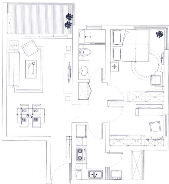
● 平面布置图
