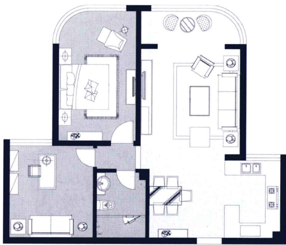
● 平面布置图
