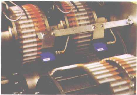
卷接生产线
