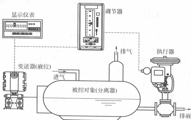
图 1-3 简单液位控制系统组成示意图
