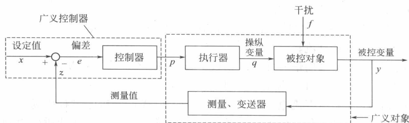
图 1-4 自动控制系统方块图
