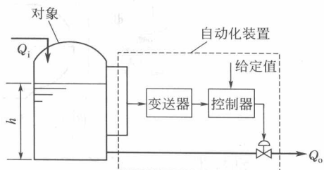
图 1-2 液位自动控制
