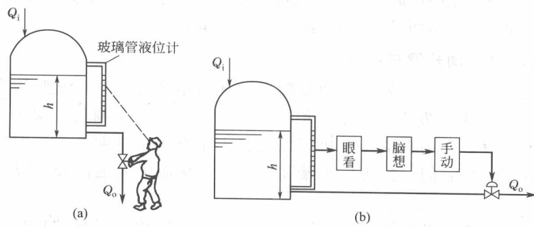
图 1-1 液位人工控制
