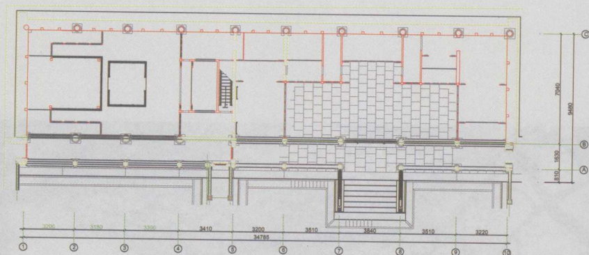
倦勤斋一层平面图
