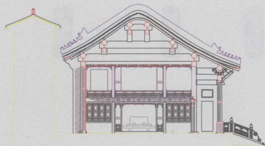
西第三间东视面
