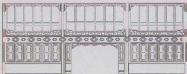
倦勤斋明间仙楼图
