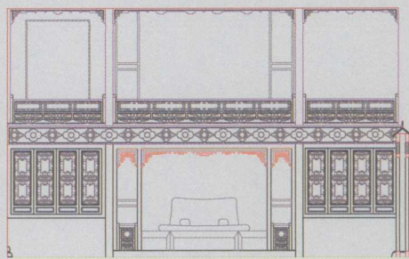
戏台东侧仙楼立面图
