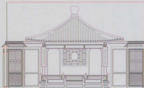
戏台立面图
