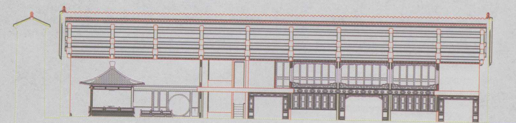
倦勤斋纵面剖面图
