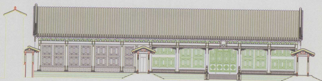
倦勤斋纵面剖面图
