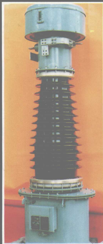
江西互感器厂生产 的油浸电流互感器
