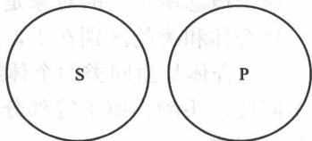
图 1-4 全异关系欧拉图
