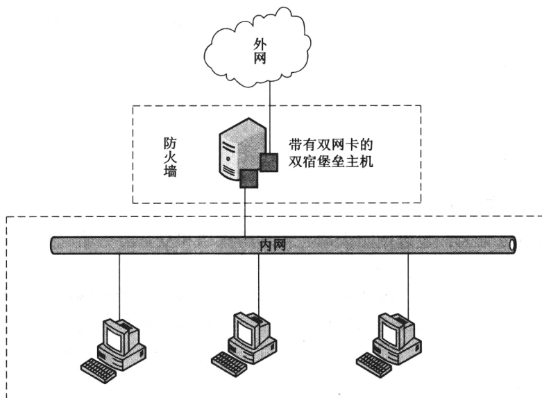
图 1-3 双宿主机结构防火墙
