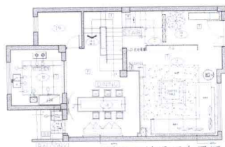
别墅二层平面布置图
