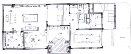
地下室平面布置图
