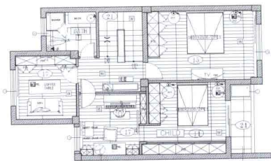
别墅三层平面布置图
