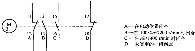
图 1.1.8 开关或触头运行方式用文字说明
