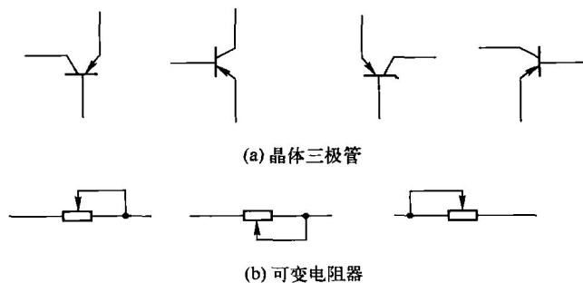
图 1.1.14 符号旋转和镜像放置示例
