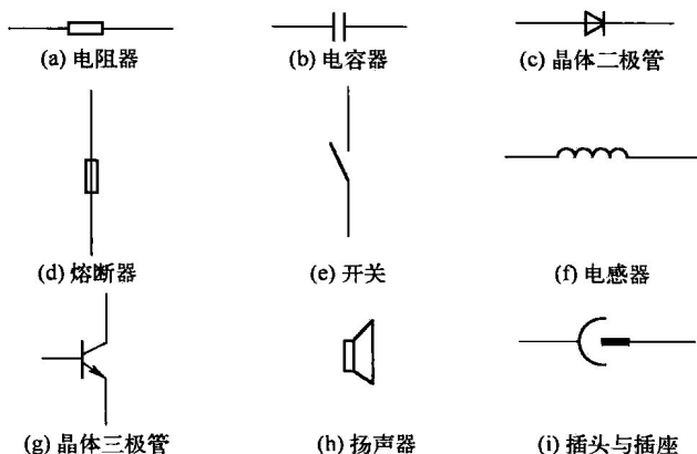
图 1.1.2 常用元器件的一般符号
