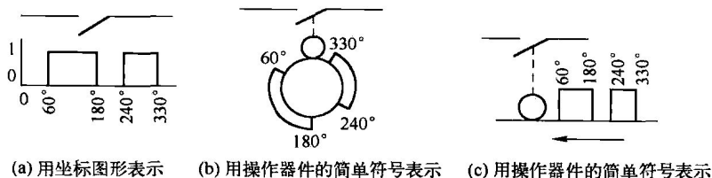
图 1.1.9 某行程开关触头位置的表示方法
