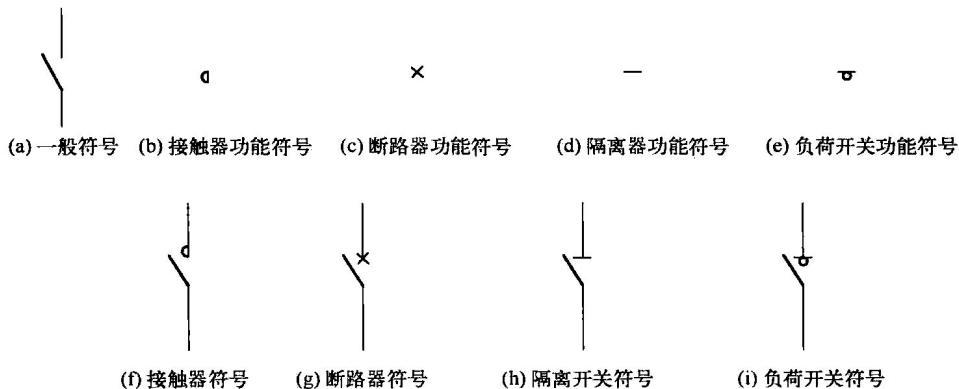
图 1.1.5 一般符号与限定符号的组合
