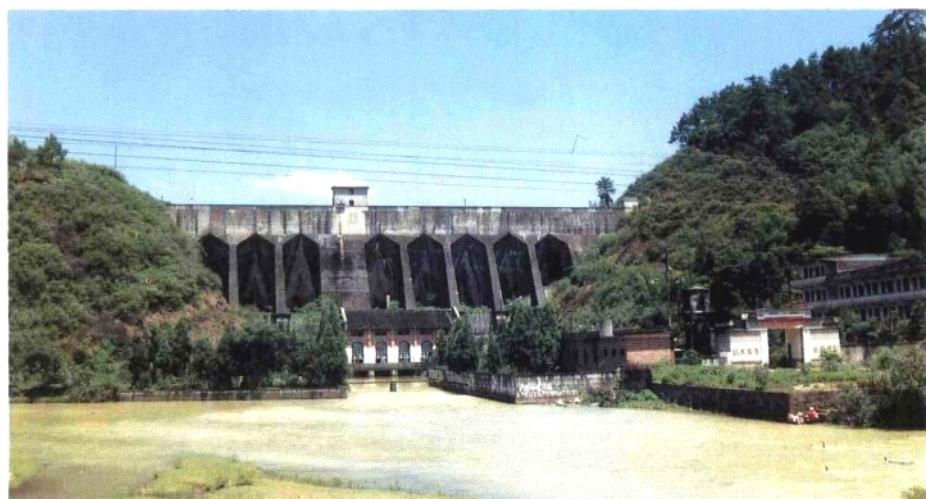
仙下水库空腹重力坝、 仙下水电站
