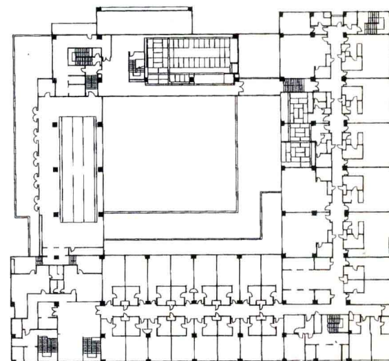
四层平面图
