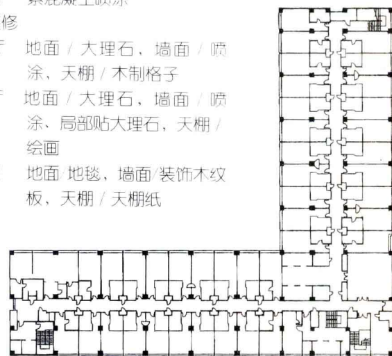
十层平面图
