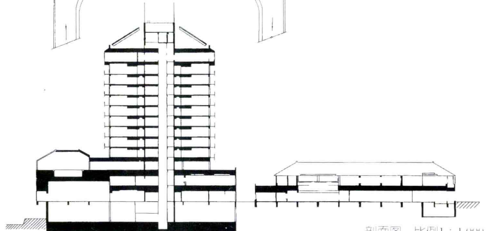
剖面图 比例1:1000
