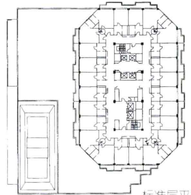
标准层平面图
