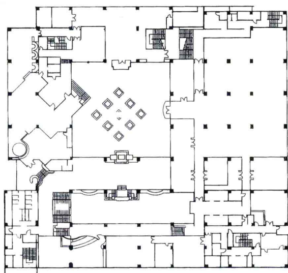
二层平面图
