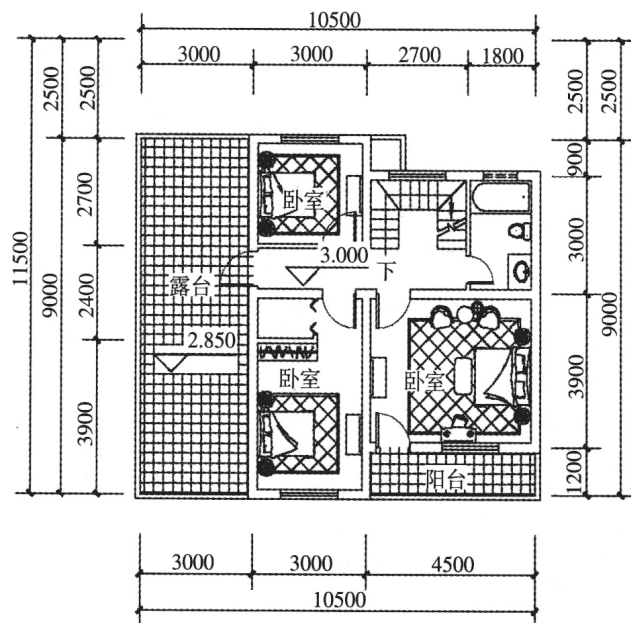
二层平面图
