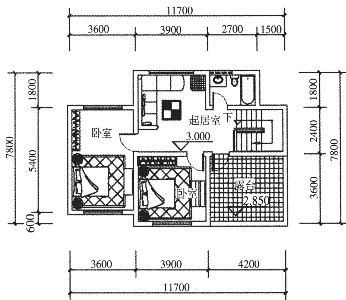
二层平面图
