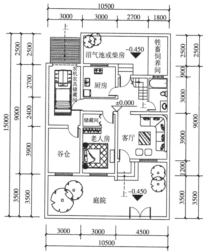
一层平面图
