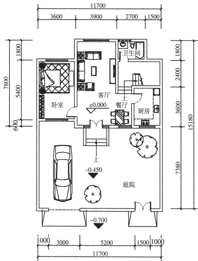
一层平面图
