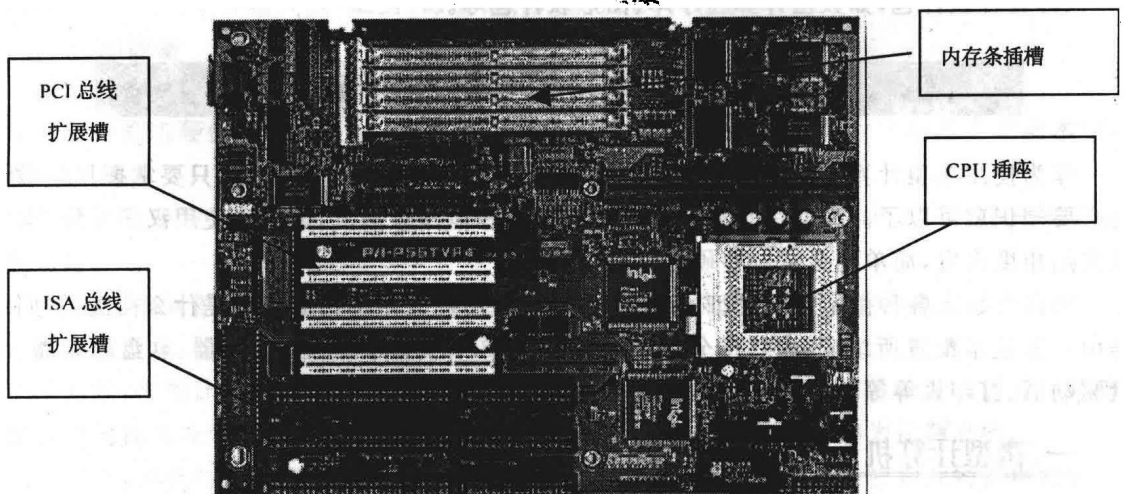
图 1.4.2 主机板示意图
